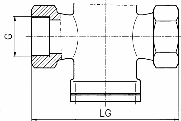
Abmessungen, Betriebsparameter / Размеры, эксплуатационные параметры
